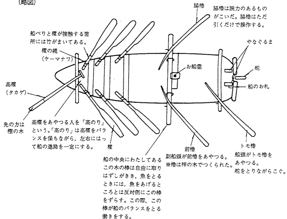
カッコ船 上から見た図 (略図)
