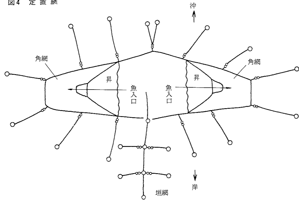
図4 定置網
