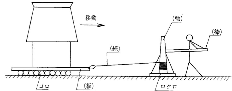
図9 コロ、ロクロによる家屋の移動略図 (佐藤久右衛門氏図示)
